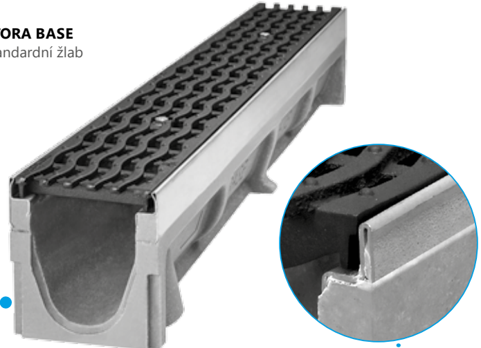
STORA BASE ochranná ocelová hrana
