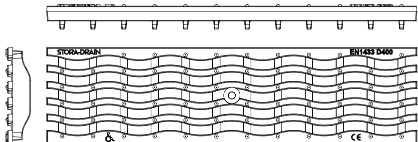
WAVE rošt z tvárné litiny
